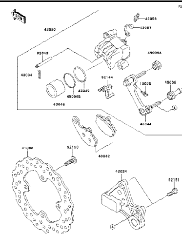
45 Rear Brake - เบรคหลัง
