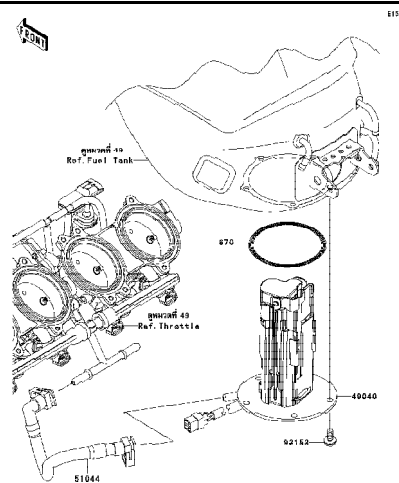
18 Fuel Pump - ปั๊มน้ำมันเชื้อเพลิง
