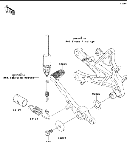
40 Brake Pedal - ค้านเหยียบเบรค
