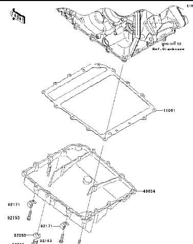
15 Oil Pan - อ่างน้ำมันเครื่อง
