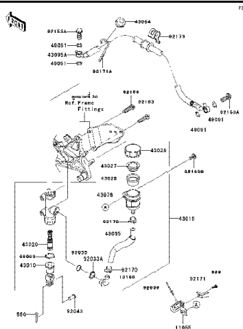
44 Rear Master Cylinder - แม่ปั้มเบรคหลัง
