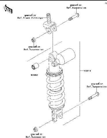
41 Shock Absorber(s) - โช้คอัพหลัง
