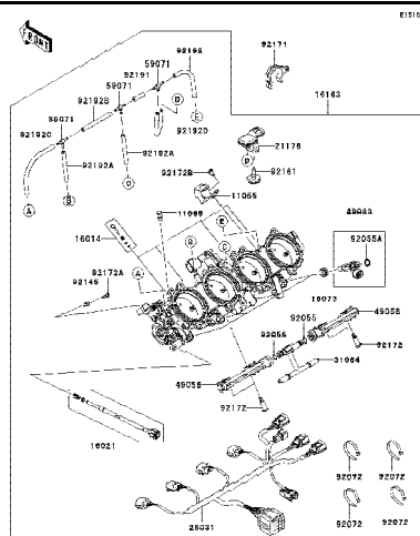
16 Throttle - ชุดลิ้นปีกผีเสื้อ
