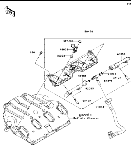
17 Top Feed Injector - ท่อน้ำมันหัวฉีด
