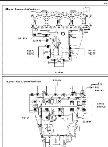
13 Crankcase Bolt Pattern - แบบแสดงตำแหน่งโบลท์เครื่องรถยนต์
