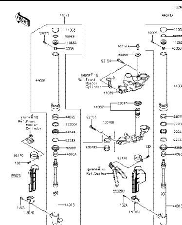
16 Front Fork - ใช้ค้ำพหน้า
