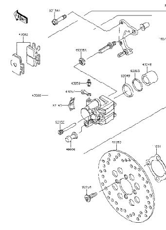
13 Front Brake - เบรคหน้า
