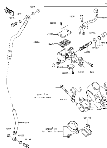
12 Front Master Cylinder - แม่ปั้มเบรคหน้า
