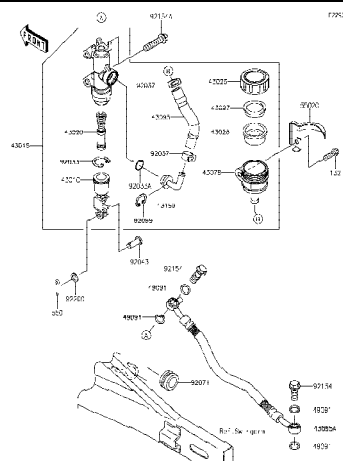
14 Rear Master Cylinder - แม่ปั้มเบรคหลัง
