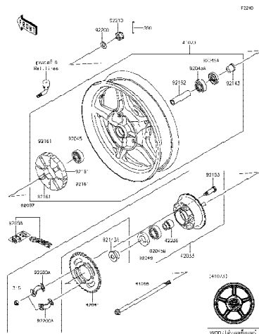
11 Rear Hub - ดุมล้อหลัง
