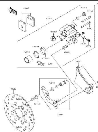
15 Rear Brake - เบรคหลัง
