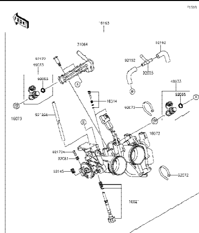
16 Throttle - ชุดลิ้นเร่ง
