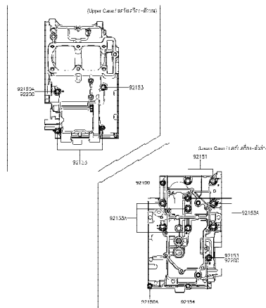
14 Crankcase Bolt Pattern - แบบแสดงตำแหน่งโบลท์แคว้งเครื่องยนต์
