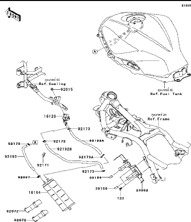
19 Fuel Evaporative System-ระบบควบคุมไอน้ำมันเชื้อเพลิง
