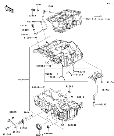
13 Crankcase-เครื่องเครื่องยนต์
