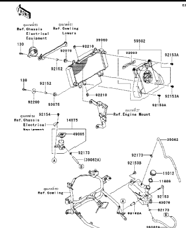
24 Radiator-หม้อน้ำ
