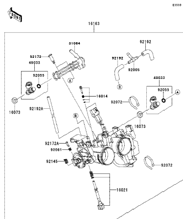
16 Throttle-ทดลึ้นเร่ง
