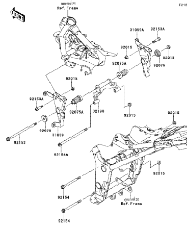
27 Engine Mount-ส่วนประกอบการยึดเครื่องยนต์
