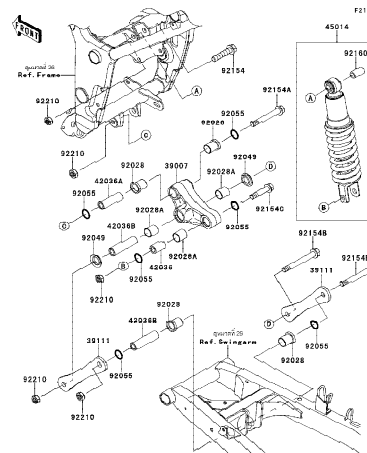
30 Suspension/Shock Absorber-โช๊คอัพหลัง
