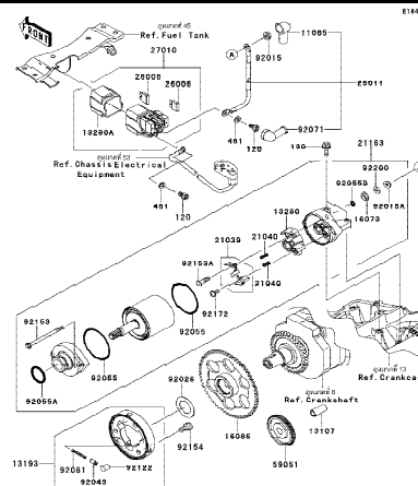
23 Starter Motor-มอเตอร์สตาร์ท
