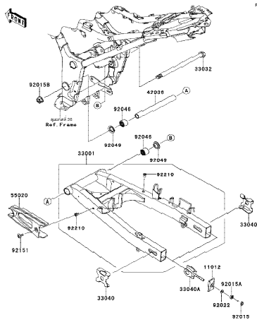
29 Swingarm-สวิงอาร์ม
