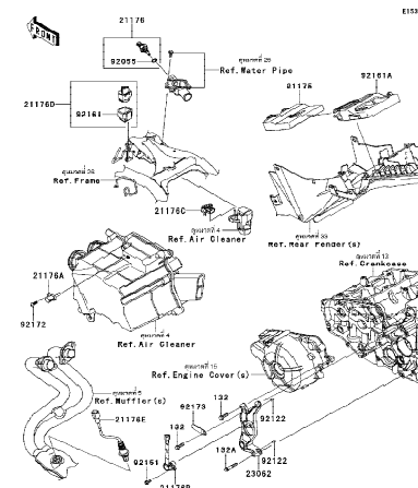
18 Fuel Injection-ตัววัดและส่งสัญญาณ
