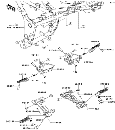
31 Footrests-พนักเท้า
