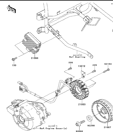
21 Generator-แม็กนีโต
