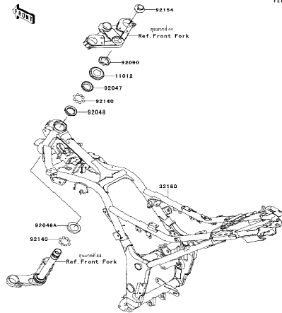
26 Frame-เฟรม
