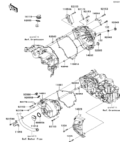
15 Engine Cover(s)-ฝาครอบเครื่องยนต์
