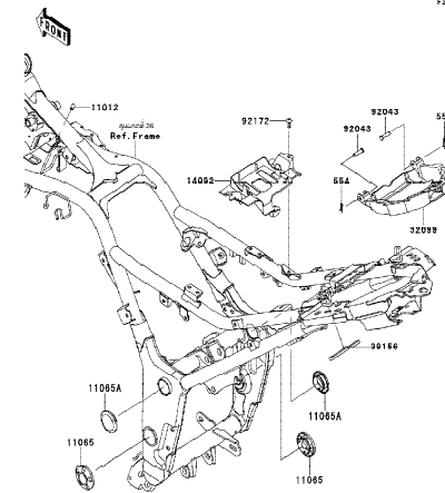
28 Frame Fittings-ส่วนประกอบการยึดกับเฟรม
