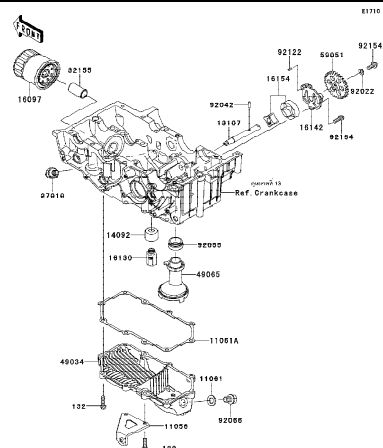
20 Oil Pump-ปั้มน้ำมันเครื่อง
