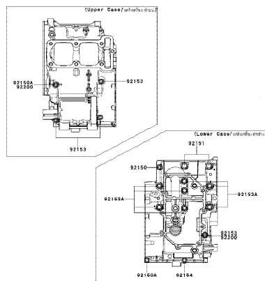
14 Crankcase Bolt Pattern-แบบแสดงตำแหน่งโบลท์เครื่องยนด
