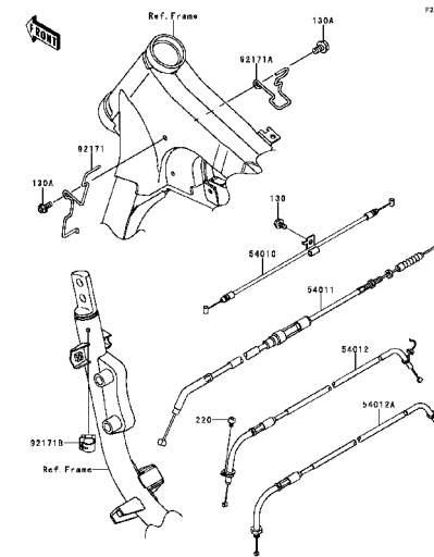
F-14 Cables
