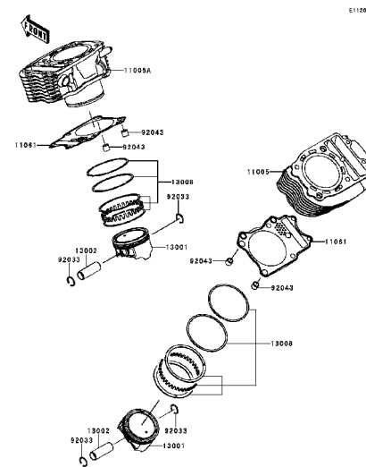
B-5 Cylinder/Piston(s)
