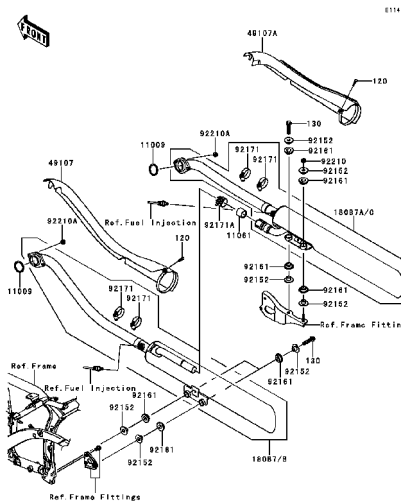
B-7 Muffler(s)
